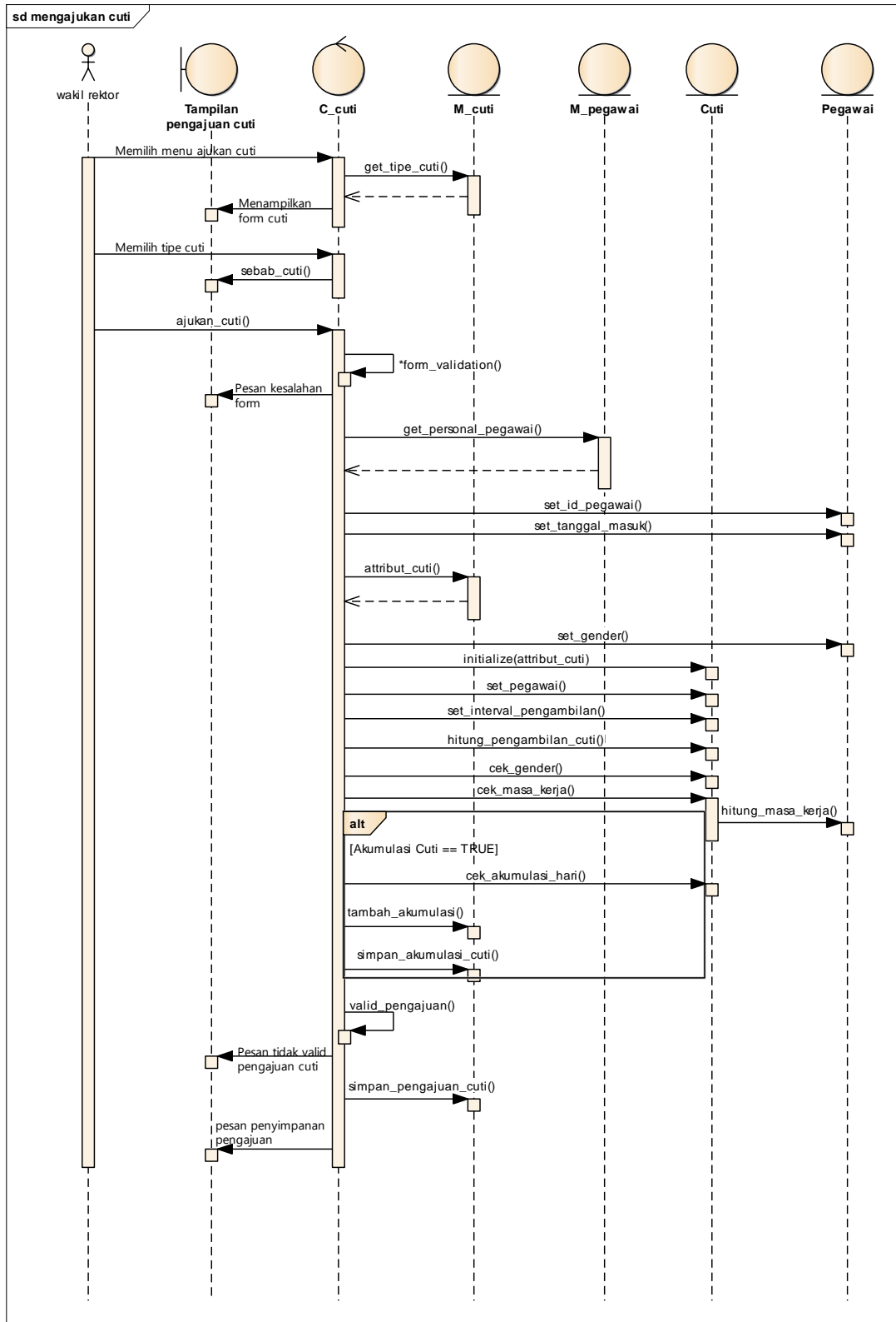
Lampiran 5. Sequence diagram wakil rektor mengajukan cuti
