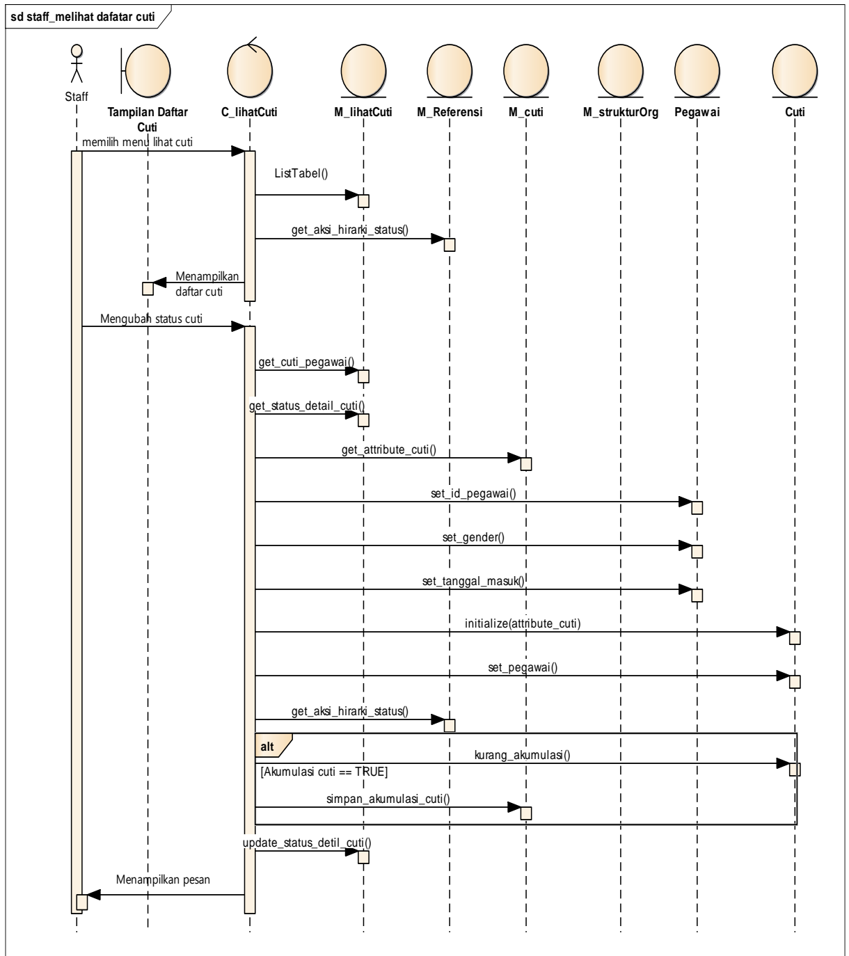
Lampiran 6. Sequence diagram staff melihat daftar dan mengubah status cuti
