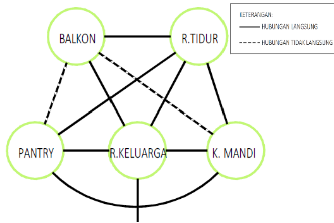
Gambar 5.3 Hubungan Ruang Tipe 1 Kamar Tidur
