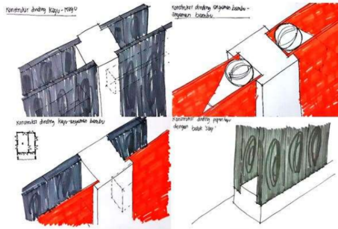
Gambar 2. Tipe konstruksi dinding pada bangunan
