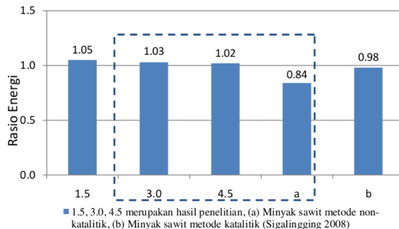
Gambar 3. Perbandingan rasio energi hasil penelitian penulis dan Sigalingging (2008) berdasarkan definisi RE_2 pada persamaan (2)
