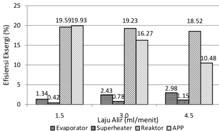
Gambar 5. Efisiensi eksergi setiap subsistem pada produksi biodiesel secara non-katalitik.
