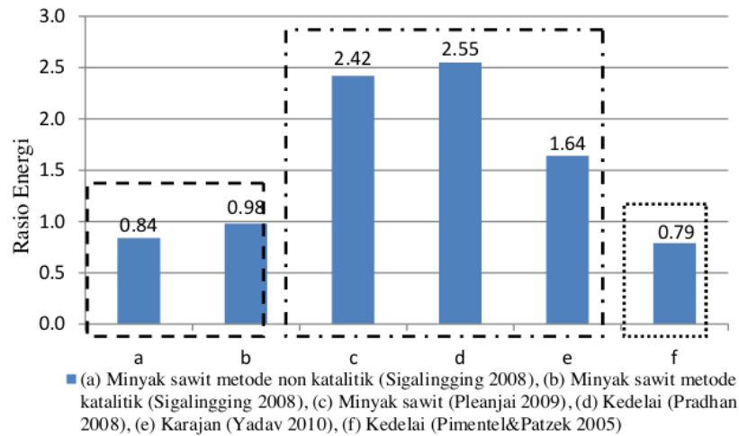
Gambar4. Perbandingan rasio energi dengan definisi yang berbeda dari berbagai literatur
