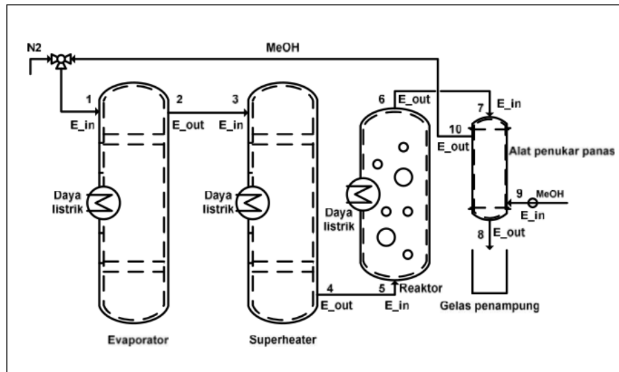
Gambar 1. Skema dan batasan alat produksi biodiesel secara non-katalitik dengan sirkulasi panas.
