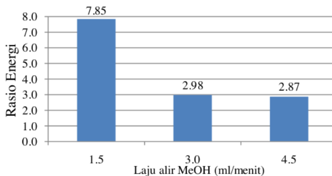
Gambar 2. Rasio energi hasil penelitian berdasarkan definisi RE_1
