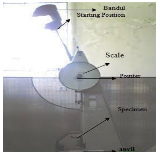
Gambar 3.8. Alat Uji Impact (Charpy)
