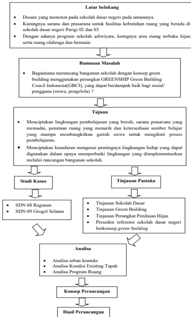
Gambar 4. Kerangka Berfikir
