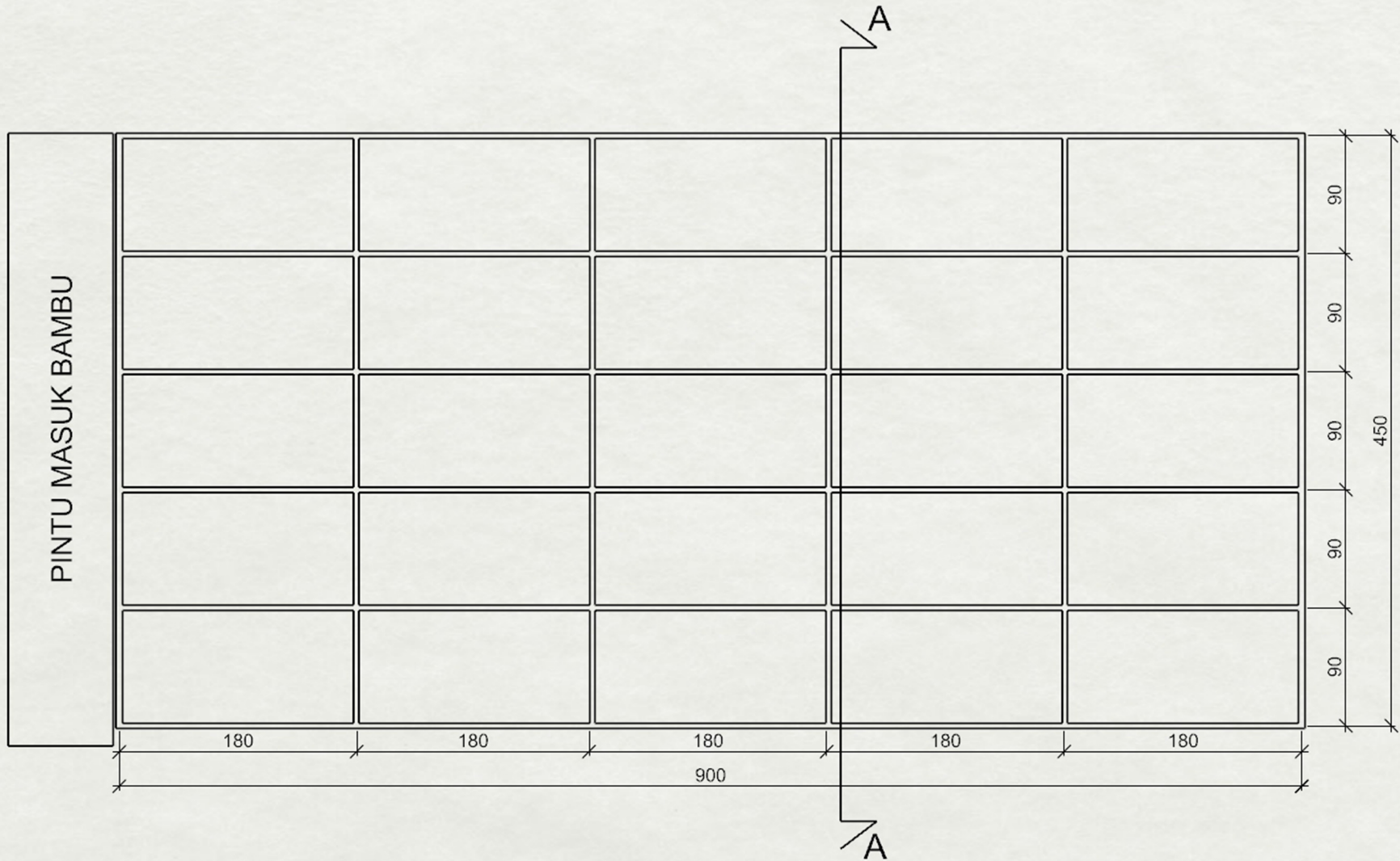
○ TAMPAK ATAS
