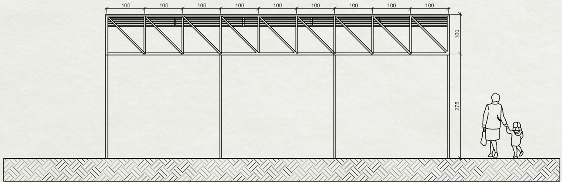
○ TAMPAK DEPAN
