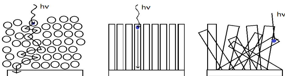
Gambar 3. Transport elektron dan penyerapan foton pada morfologi bentuk film \text{TiO}_2 nanopartikel (a) dibandingkan dengan morfologi \text{TiO}_2 nanotube non array (b) dan morfologi TNTAs (c)
