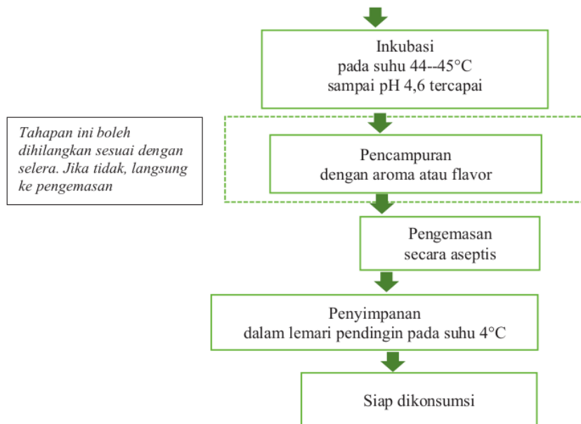
Gambar 1. Proses produksi yoghurt
