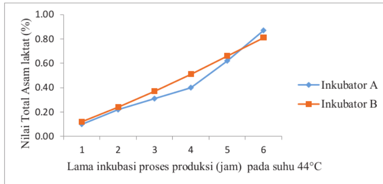
Gambar 7. Kenaikan total asam (asam laktat) dari dua percobaan dengan bahan susu dan biang yoghurt pada inkubator A dan B
