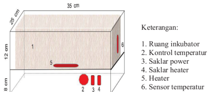
Gambar 3a: Gambar skematik inkubator
