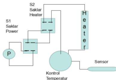
Gambar 3b: Wiring unit yang dipasang dalam inkubator
